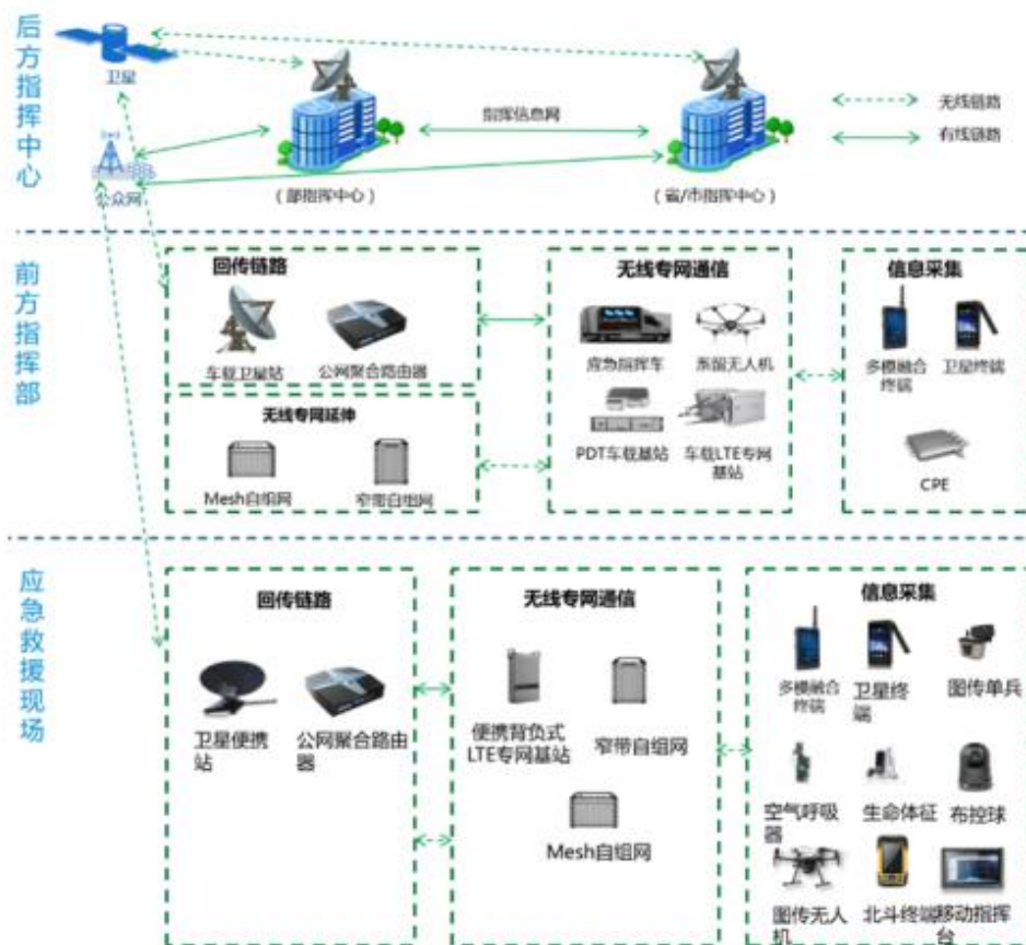
图3 应急通信总体架构图
